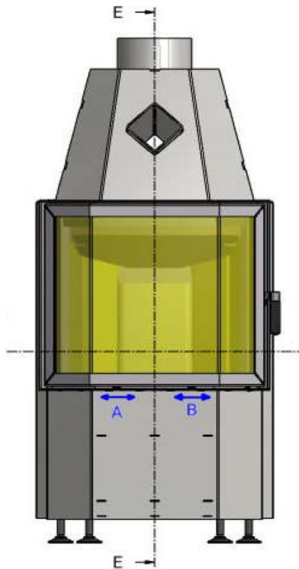
Abb. 1.6. Luftregler
